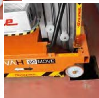
Überrollschutteinrichtung
